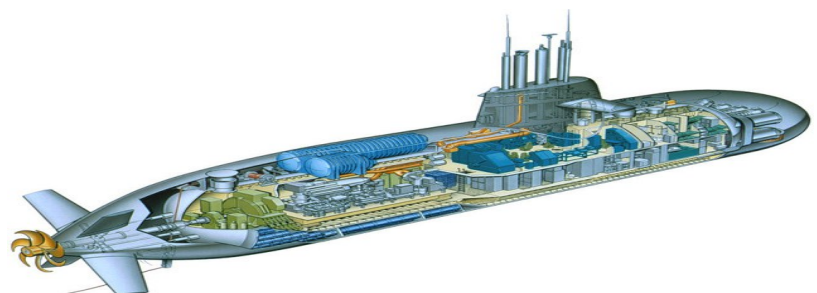
Sottomarini della classe Sauro (in alto) e Todaro (in basso).
